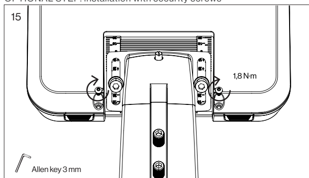
PASO OPCIONAL: instalación con tornillos de seguridad OPTIONAL STEP: installation with security screws
